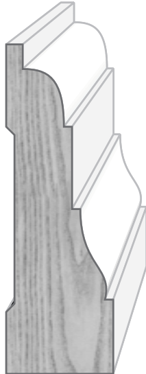
RWCA-02 13/16" X 2-1/2"
