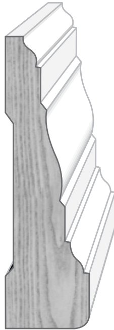
RWCA-08 7/8" X 3"
